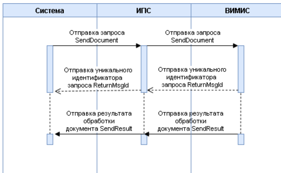
Рисунок 2 – Общая схема взаимодействия Системы, ИПС ЕГИСЗ и ВИМИС «СЗ»
